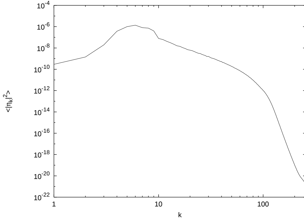
Рис. 4.20: Корреляционная функция отклонения поверхности в двойном логарифмическом масштабе.
