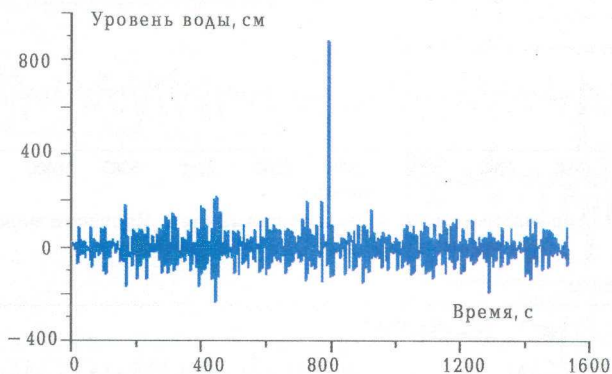
Рис. 1.10. Аномальная волна, зарегистрированная с буя в Черном море 22 ноября 2001 г. [12, 30]
